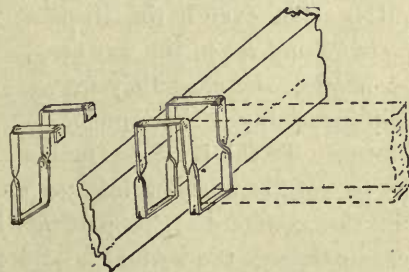
FIG. 24—STIRRUP IRONS.
